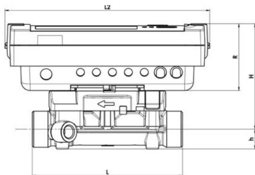
Dimensions de l'électronique L2 x B x R = 150 x 100 x 50 mm
